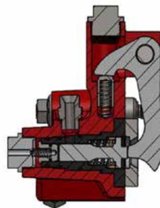
SECTION A-A SCALE 1 : 3
